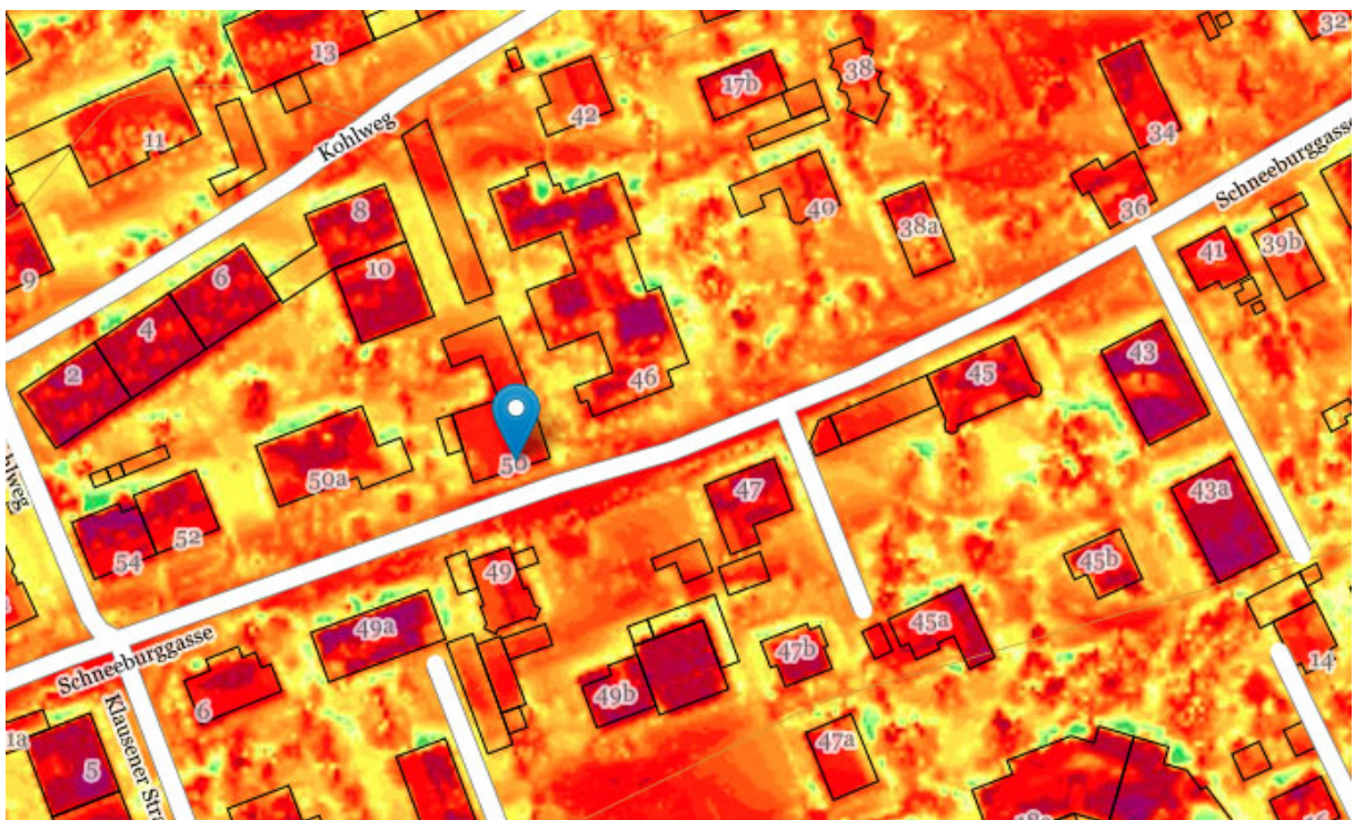
Sonnenscheindauer 21. Jun
