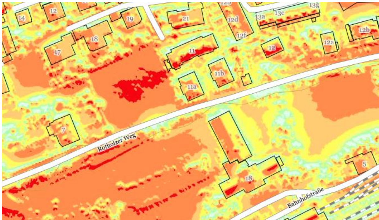
Solarstrahlung Jahr
