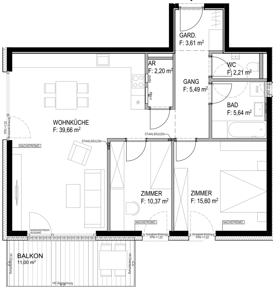
AW 04 84,78 m 2
