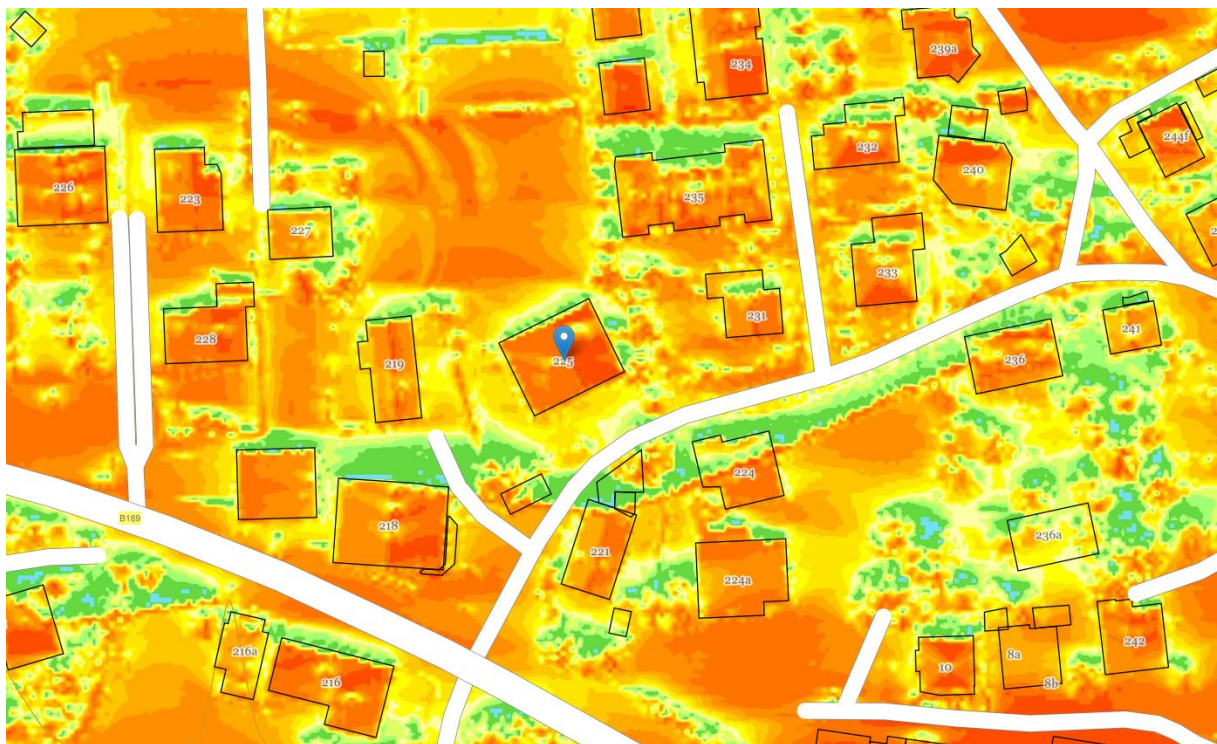
Sonnenscheindauer 21. März
