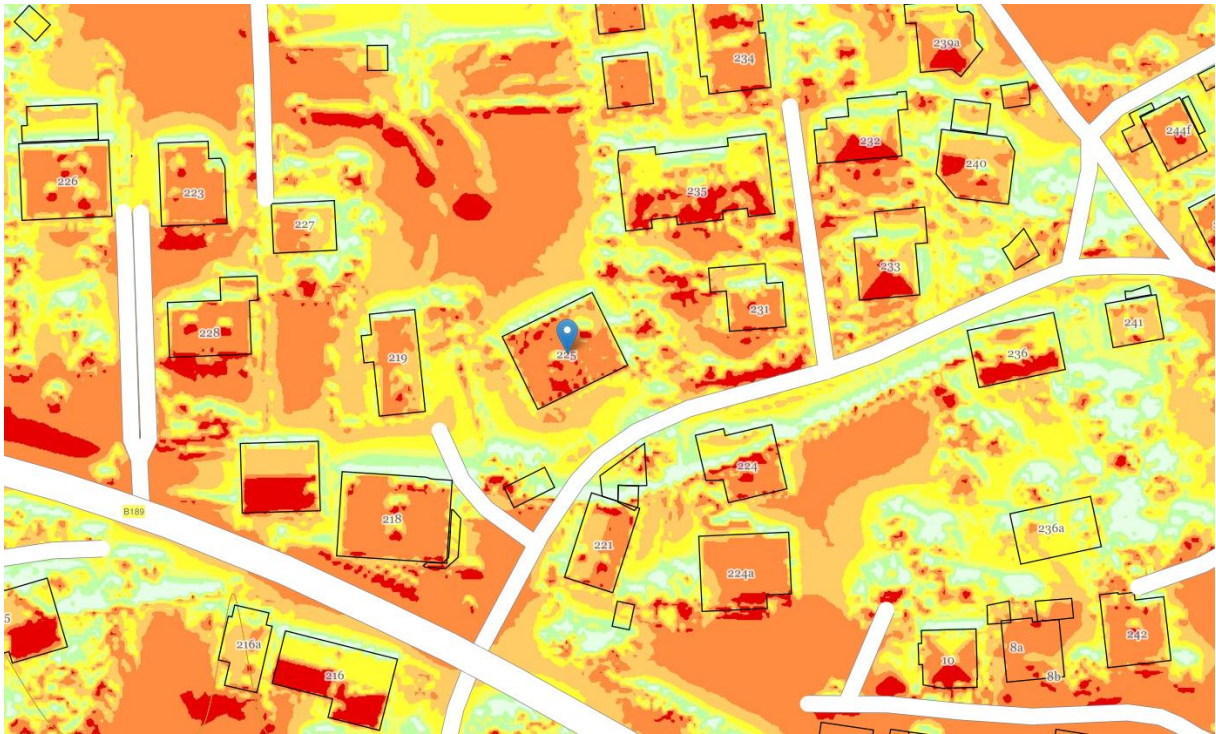
Solarstrahlung Jahr
