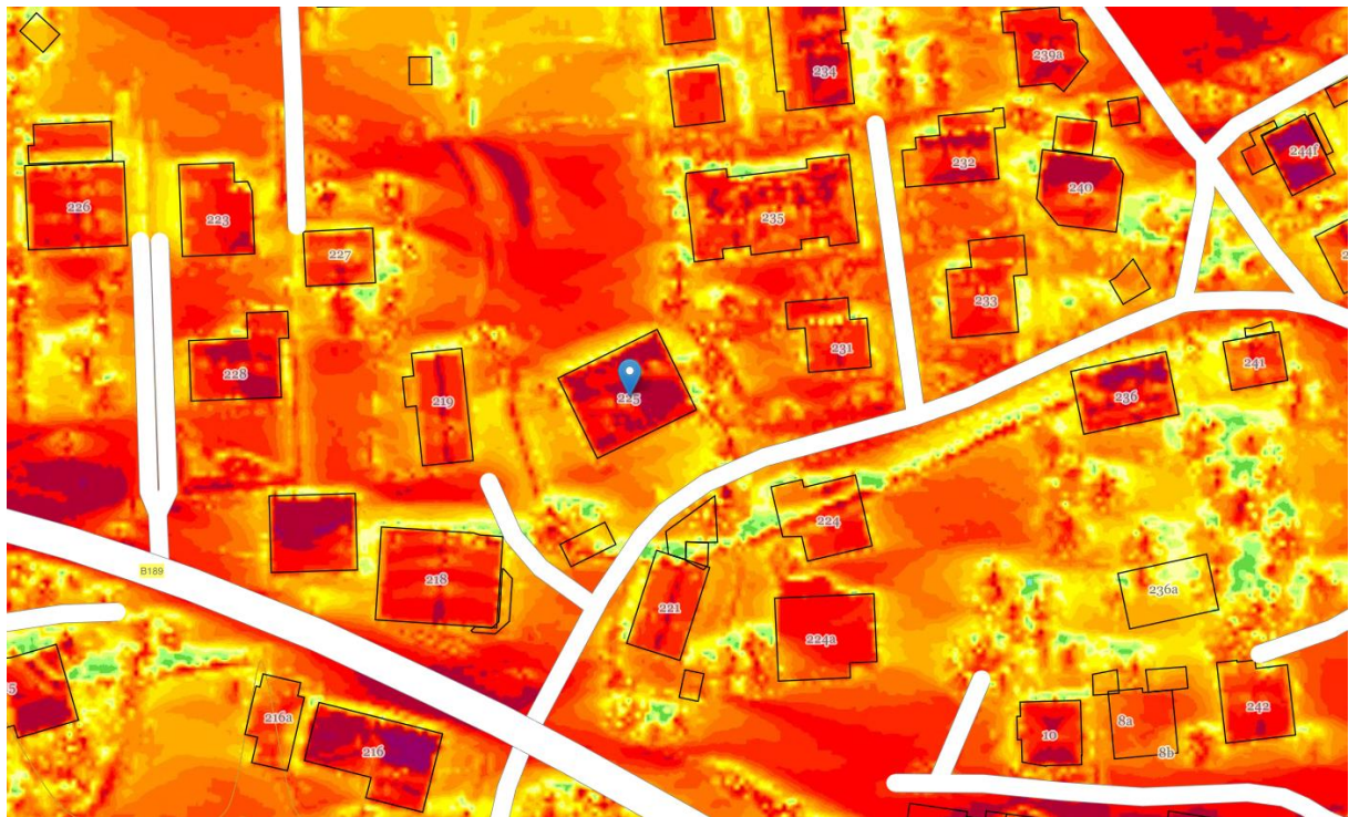
Sonnenscheindauer 21. Mai
