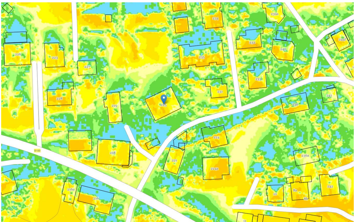
Sonnenscheindauer 21. Dez
