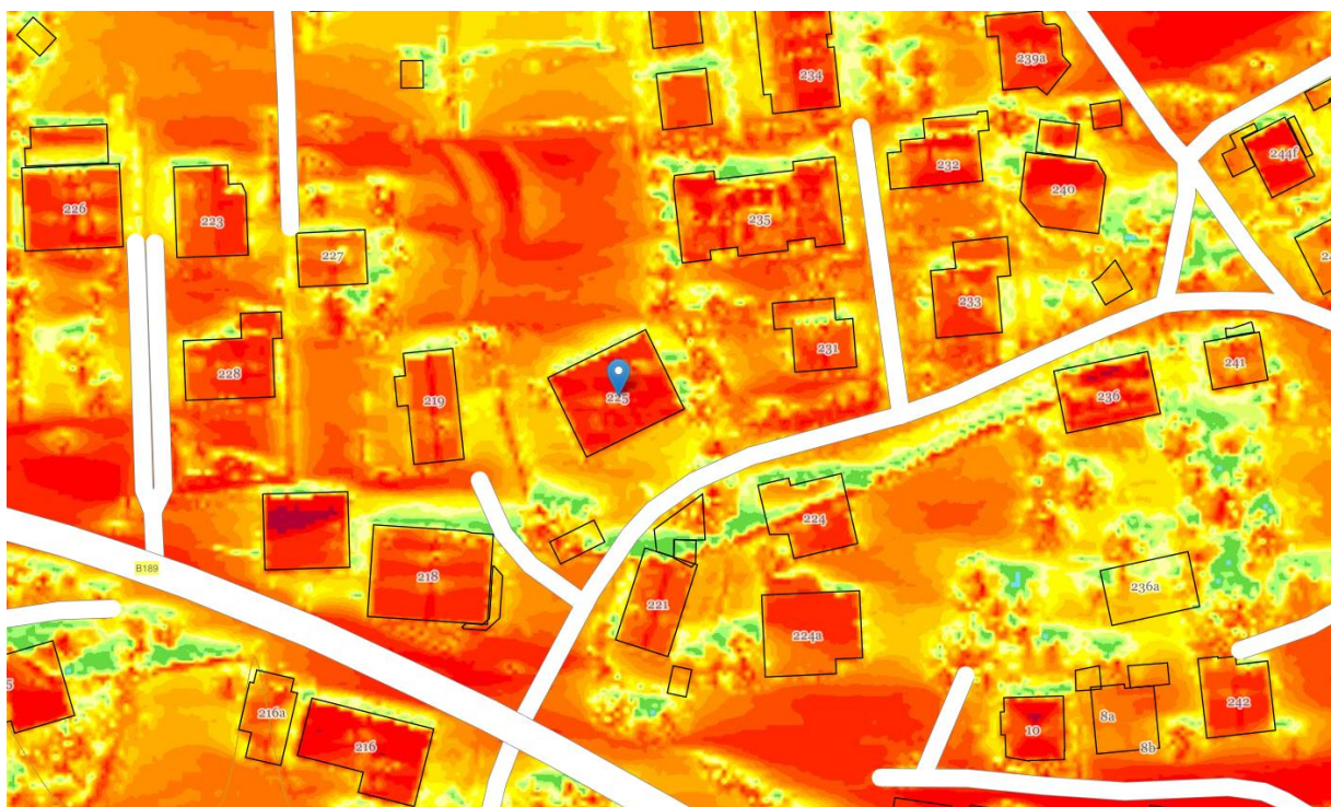
Sonnenscheindauer 21. Apr
