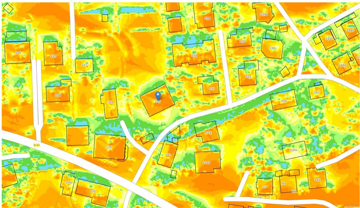
Sonnenscheindauer 21. Feb
