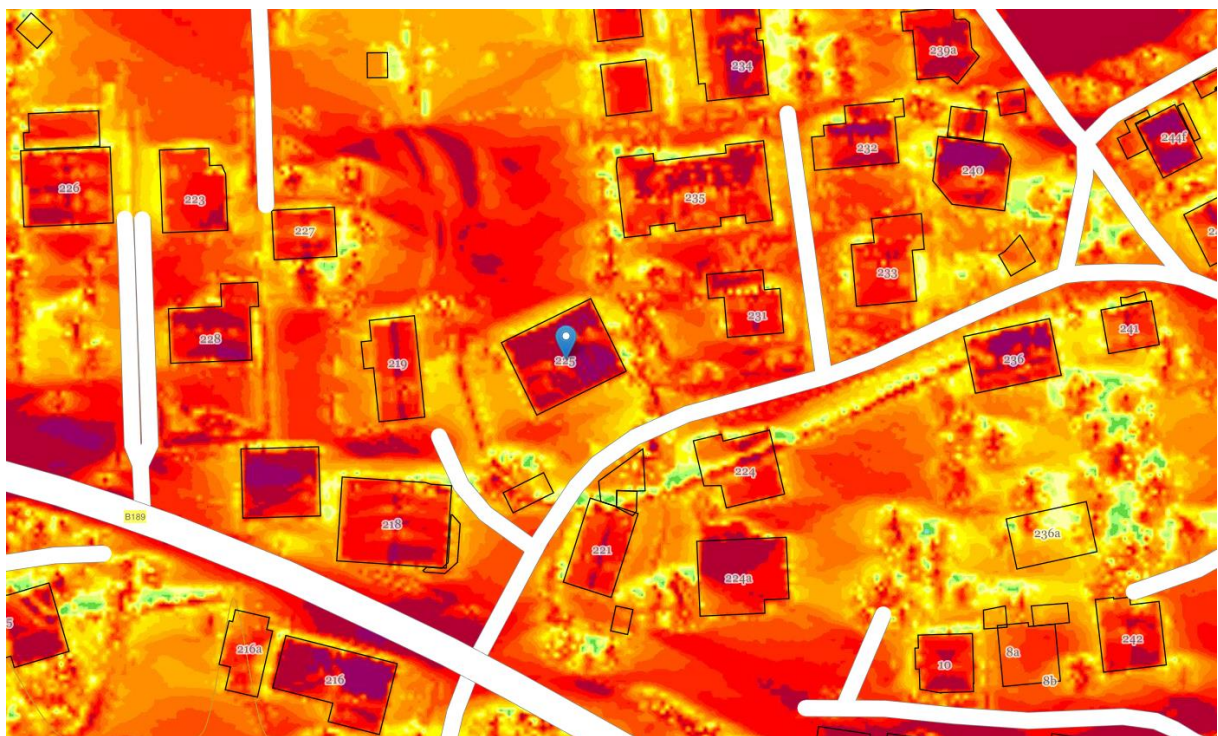
Sonnenscheindauer 21. Jun
